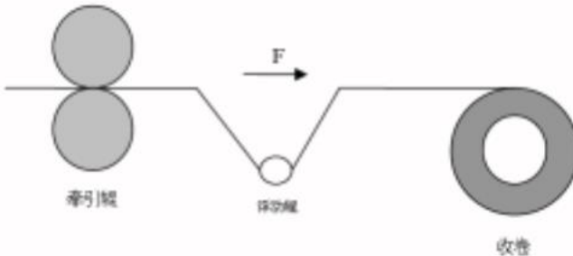
图2 带浮动辊张力反馈
