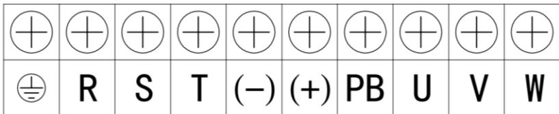
圖 3-2 三相 400V 輸入 2R2GB/4R0PB~015GB/018PB 主回路接線端子
