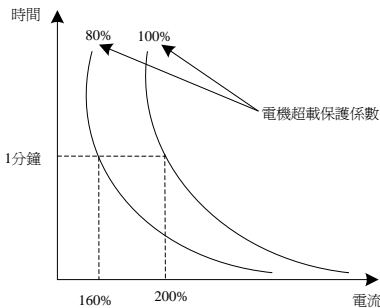
圖6-26 電機超載保護係數設定
