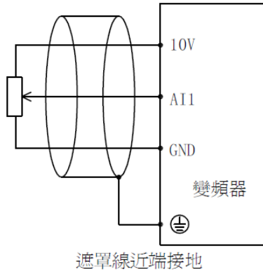
圖 3-14 類比量輸入的連接方式
