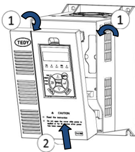
圖 2-5 下蓋板的拆卸
