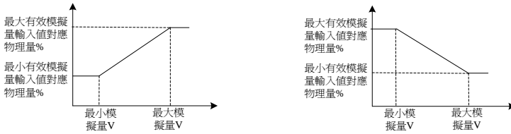
圖6-18 類比輸入線性曲線
