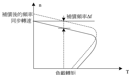
圖6-11自動轉差補償
