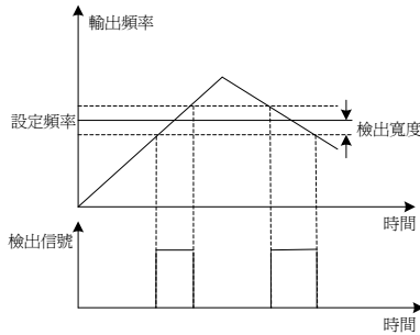
圖 6-19 頻率到達檢出寬度示意圖
