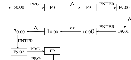
圖 4-2 三級功能表操作流程圖
