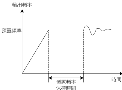
圖 6-23 預置頻率保持示意圖
