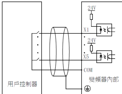
圖 3-10 控制回路端子接線說明
