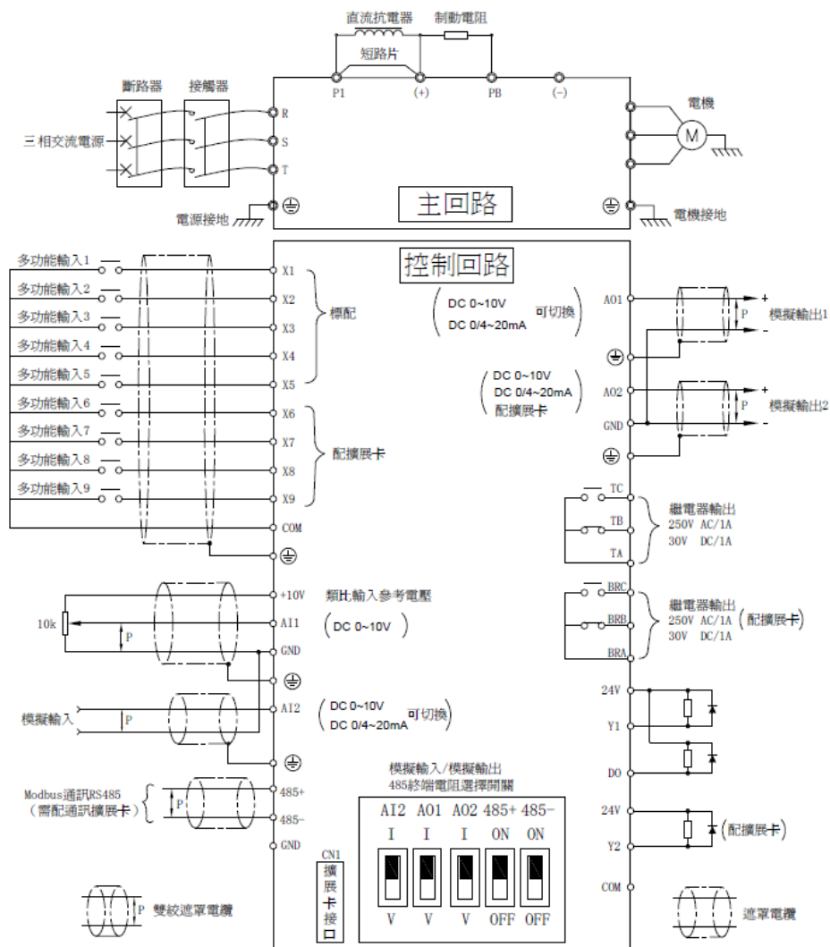
圖 3-8 端子配線圖 (以 DY300-T4018G/022P 及以上型舉例)
