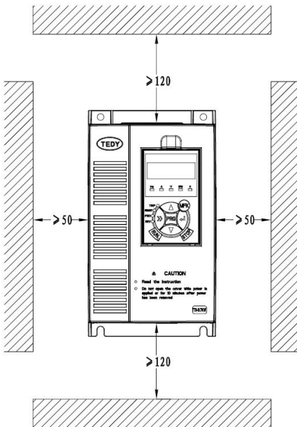
圖 2-1 DY300 安裝方向和空間
