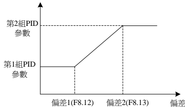
圖 6-22 PID 參數自動切換
