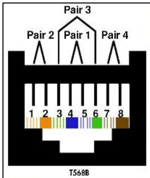
圖 3-15 T568B 標準
