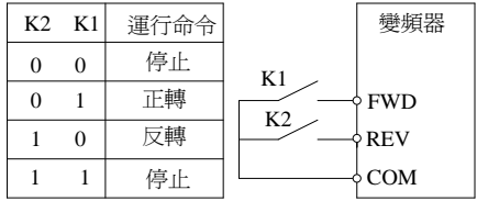
圖 6-13 兩線式 1
