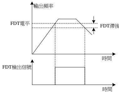
圖6-20 FDT電平示意圖
