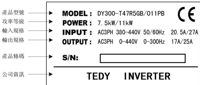
圖 1-2 產品銘牌說明
