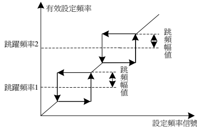
圖6-5 跳躍頻率
