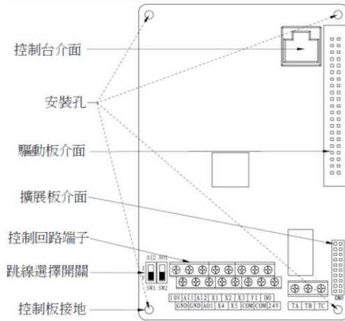
圖 3-16 控制板示意圖
