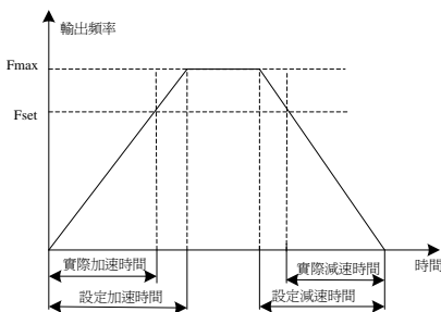
圖6-2 加減速時間示意圖
