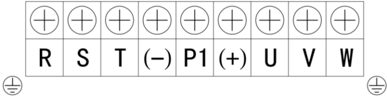
圖 3-3 三相 400V 輸入 018G/022P-110G/132P 主回路接線端子
