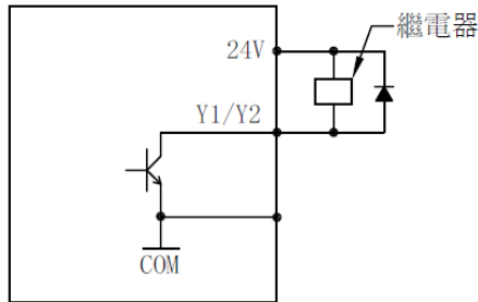
圖 3-12 內部 24V 電源連接方式
