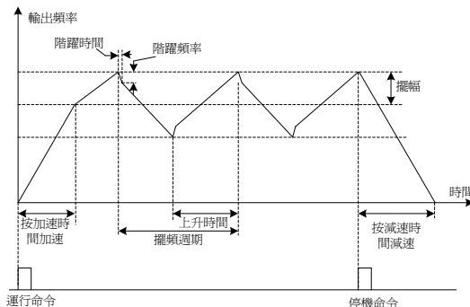
圖6-25 擺頻運行示意圖
