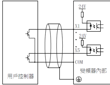
圖 3-11 NPN 型共發射極連接方式
