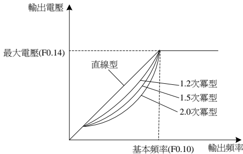
圖6-8 V/F曲線示意圖
