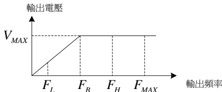
圖6-1 輸出頻率與輸出電壓關係圖
