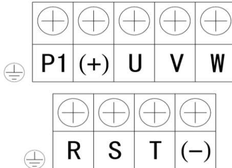
圖 3-4 三相 400V 輸入 160G/200P-500G/560P 主回路接線端子
