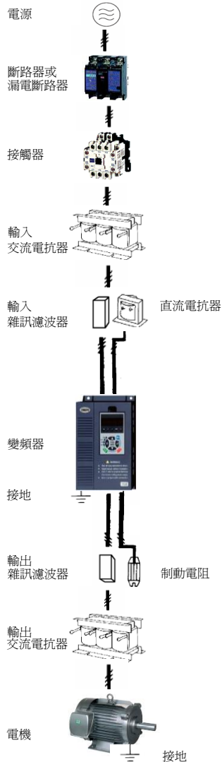
圖 3-1 產品與週邊器件的连接圖
