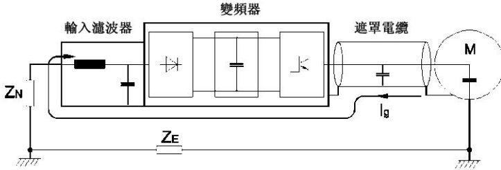
圖 3-6 傳導和輻射干擾的對策
