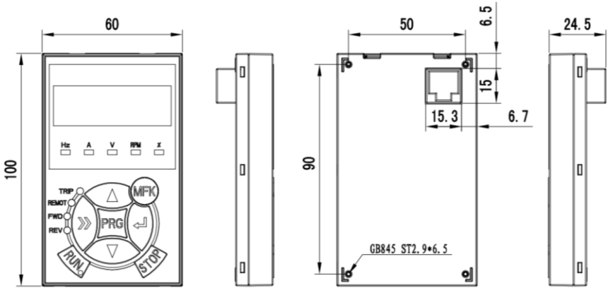
圖 1-4 操作面板的外形和安裝尺寸
