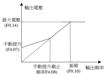
圖6-10 轉矩提升
