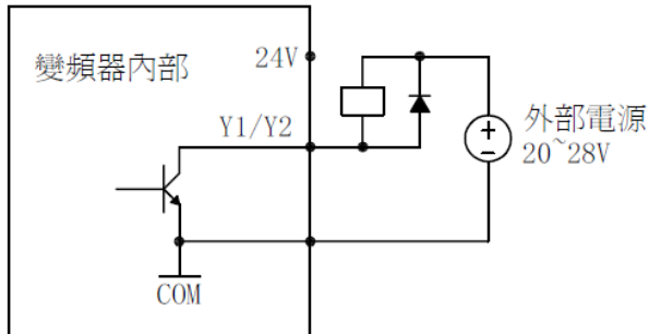
圖 3-13 外部電源連接方式
