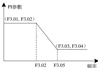
圖6-7 速度環PI參數示意圖
