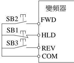
圖6-15 三線式1
