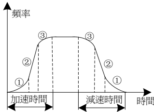
圖6-4 S曲線加減速
