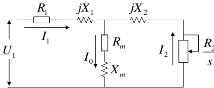
圖6-12 非同步電機穩態等效電路圖
