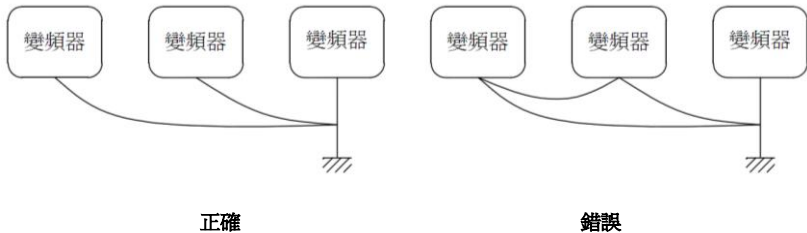
圖 3-5 接地線配線
