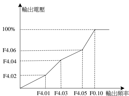
圖 6-9 多點 V/F 曲線
