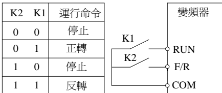
圖 6-14 兩線式 2
