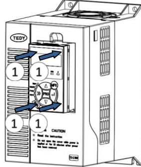
圖 2-4 操作面板的安裝
