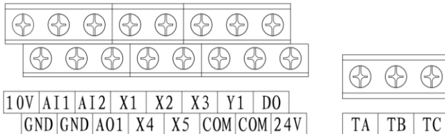
圖 3-9 標配控制回路端子排列順序
