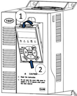
圖 2-3 操作面板的拆卸
