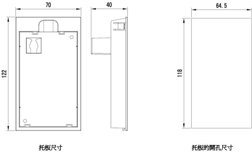
圖 1-5 托板的外形和安裝尺寸
