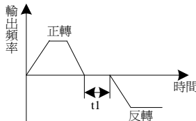
圖6-6 正反轉切換
