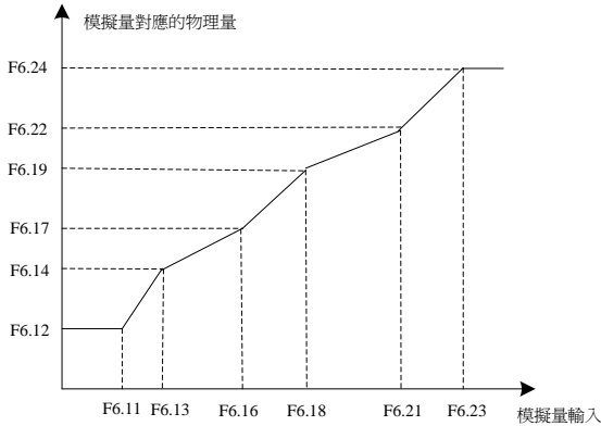
圖 6-17 類比輸入非線性曲線
