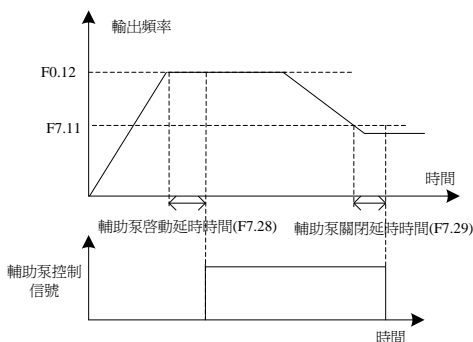
圖6-21 恒壓供水輔助泵控制信號
